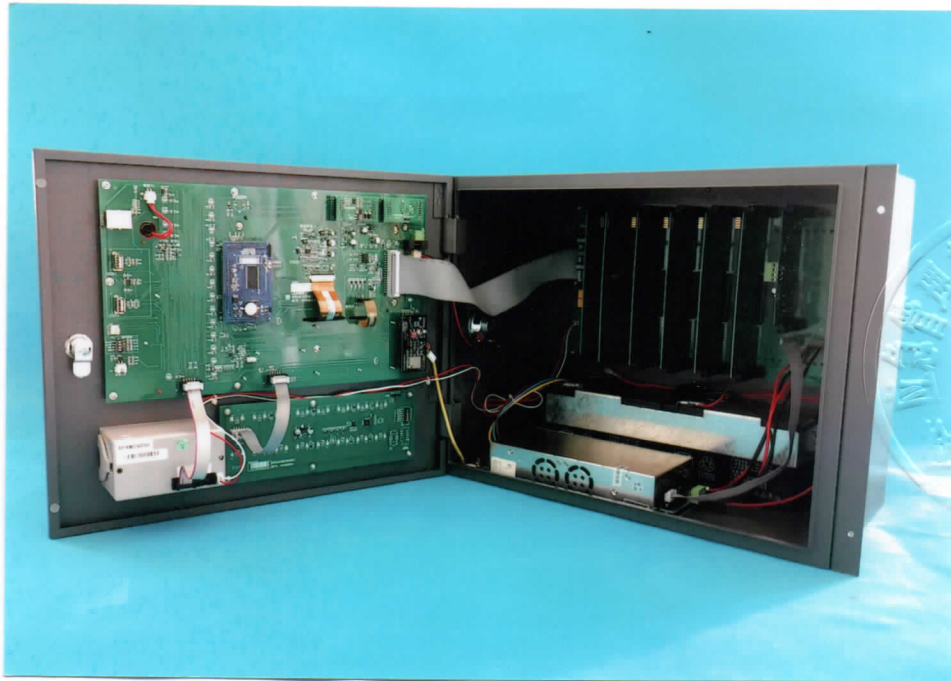
产品内部照片
