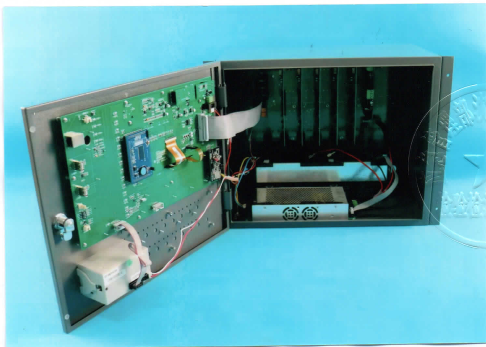
配接 YJG5211B 型电源
